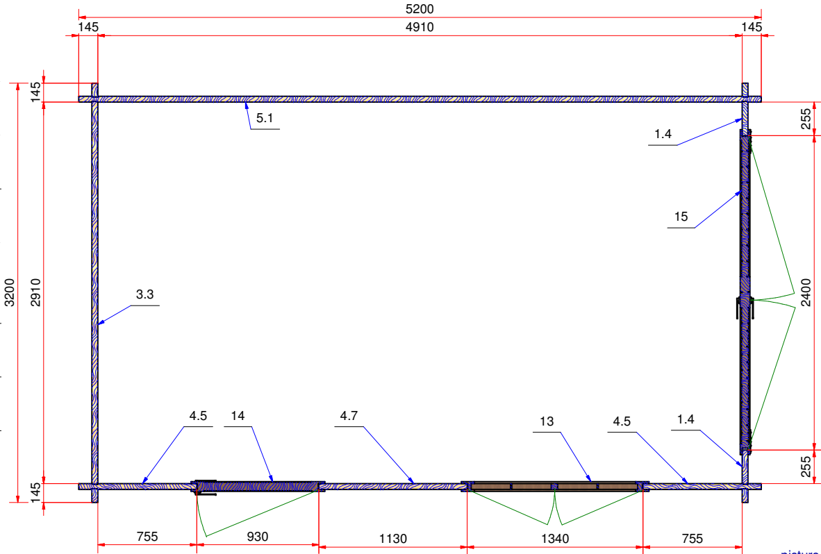
План дома (house plan)
